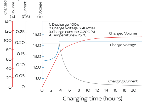
Заряд постоянным напряжением (ограничение тока 0,3С А, 25 °С)
